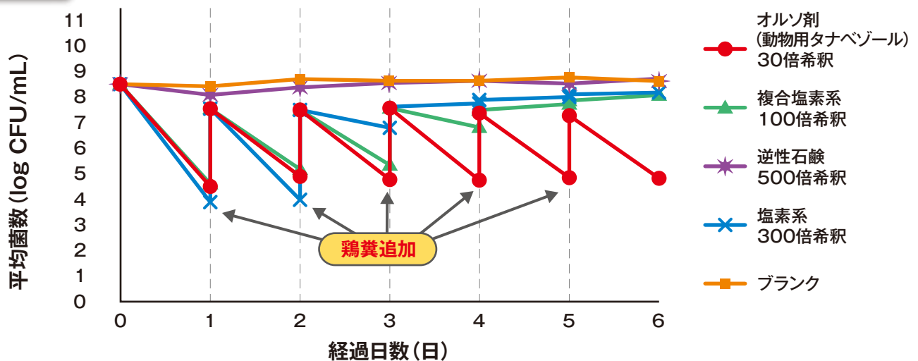
有機物存在下における各種消毒剤の総菌数の推移
